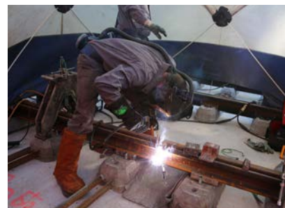
Première soudure électrique des rails du tram, une technique inédite en France
